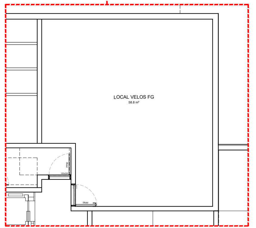
PLAN DU SOUS-SOL FG 1/500
